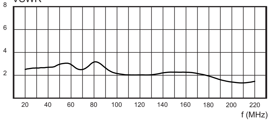
VSWR
