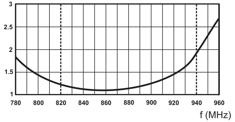
VSWR
